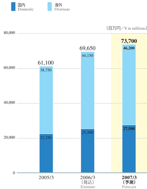
ウェハ搬送ロボット販売金額推移 Sales of wafer conveyance robots
